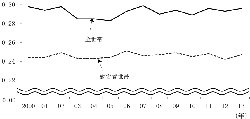
図 18-2 ジニ係数
